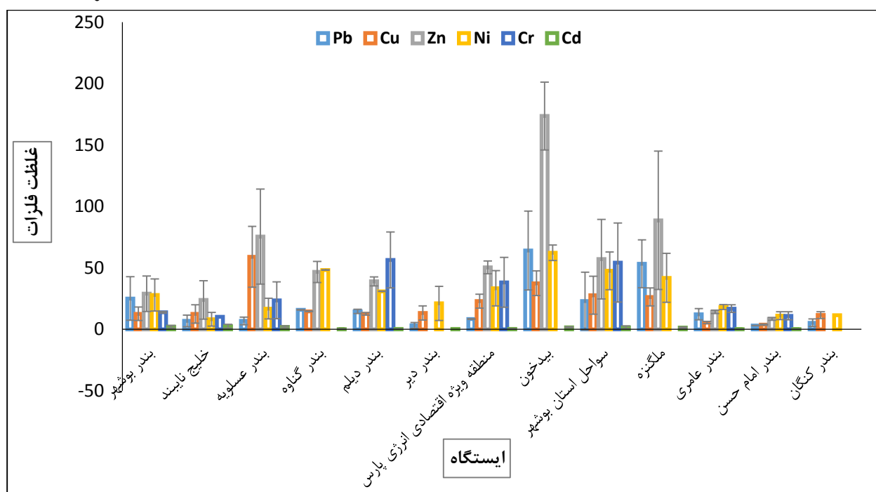
شکل ۲: مقایسه میانگین غلظت فلزات سنگین مورد بررسی در ایستگاه‌های مختلف مطالعاتی طی دوره ۱۳۹۱-۱۳۹۹
