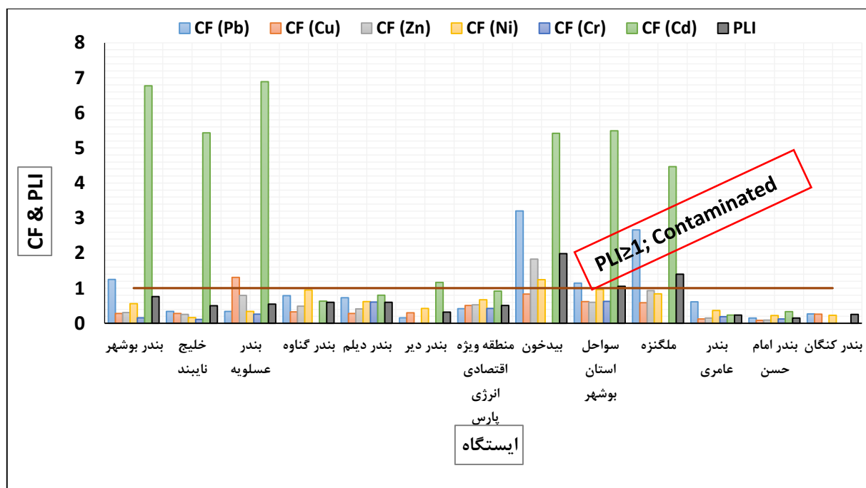
شکل ۳: میانگین فاکتور آلودگی (CF) و شاخص بار آلودگی (PLI) فلزات در ایستگاه‌های مختلف طی دوره ۱۳۹۱-۱۳۹۹
