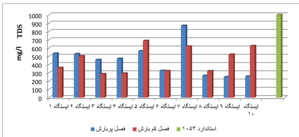
نمودار ۲: مقادیر جامدات محلول کل اندازه گیری شده منابع آب سطحی و زیرزمینی حوزه سد لثیان (سه ساله)
