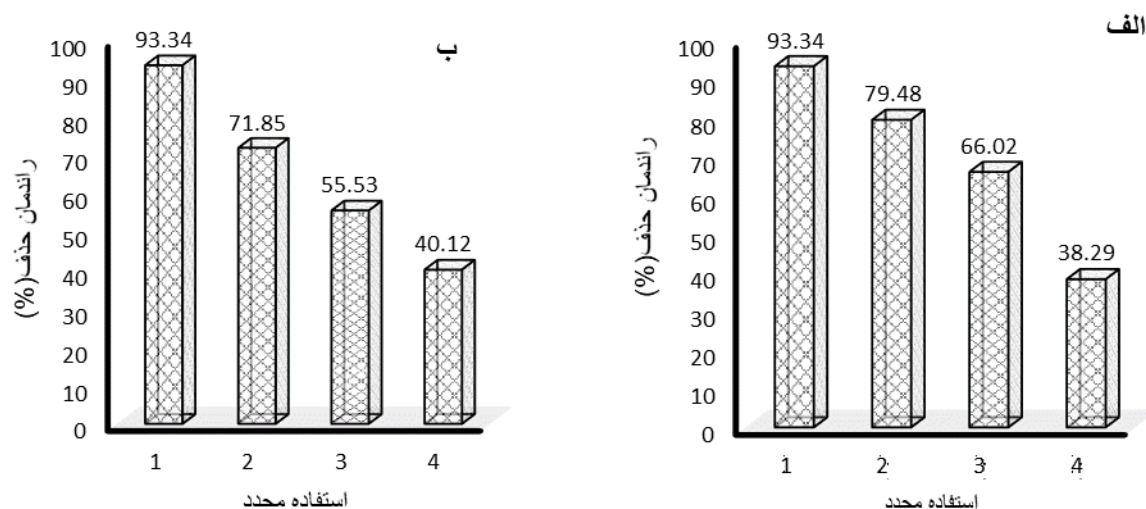
شکل ۱۱: تعیین قابلیت استفاده مجدد جاذب P_4VP - Fe_3O_4 با دو غلظت ۰.۵ g/L (الف) و ۰.۲۵ g/L (ب).
