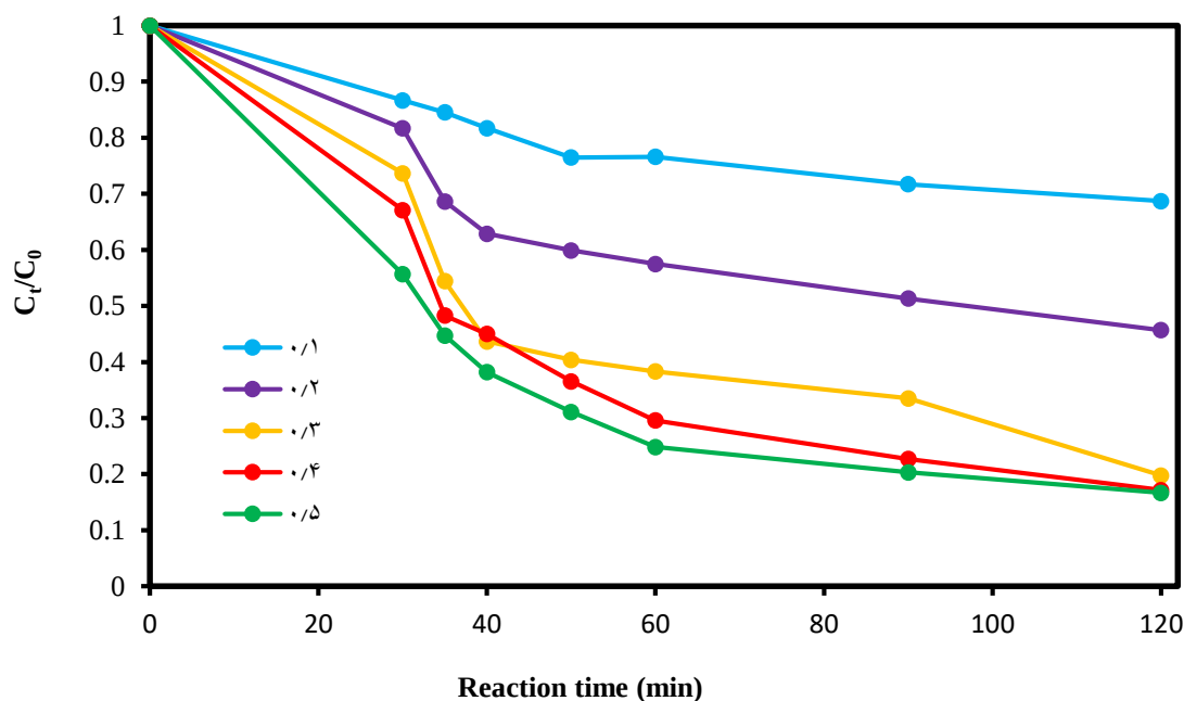
شکل ۵. تأثیر دوز کاتالیست در زمان های مختلف بر روی عملکرد فرایند MNPs-ACC/PS/UV در شرایط ثابت (غلظت اولیه بنزوتریازول: ۳۰ میلی گرم بر لیتر، غلظت پرسولفات: ۳ میلی مول و pH برابر با ۶)
