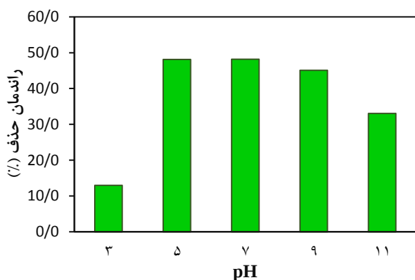
شکل ۲: اثر pH اولیه محلول بر عملکرد فرایند PMS/MnOOH. راندمان حذف ۴-کلروفنل. شرایط آزمایش: دوز PMS: ۰/۷ میلی مول، دوز MnOOH: ۰/۰۵ گرم بر لیتر، غلظت ۴-کلروفنل: ۰/۰۵ گرم بر لیتر، زمان واکنش: ۶۰ دقیقه
