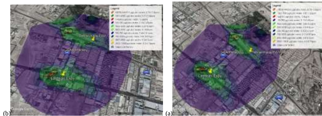
شکل ۵: نحوه پراکنش غلظت میانگین ۸ ساعته منوکسید کربن منتشر شده از کارخانه خودروسازی سایپا و بزرگراههای اطراف
