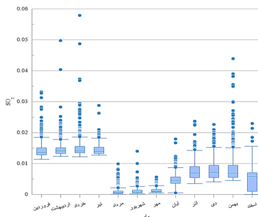
شکل ۱۶- نمودار جعبه‌ای مقادیر SO2 ثبت شده در ایستگاه فیض در سال ۱۴۰۰
