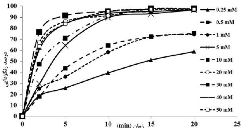
شکل ۵: اثر غلظت پراکسید هیدروژن در حضور UVC در غلظت متیلن بلو ۶ mg/L
