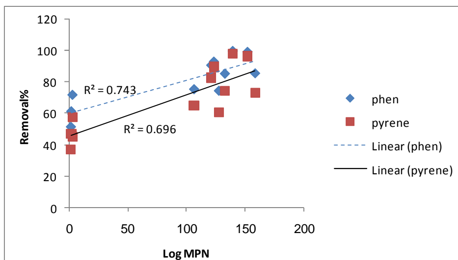
نمودار ۱: همبستگی باکتری خاک با درصد حذف فنانتروتن و پایرن خاک
