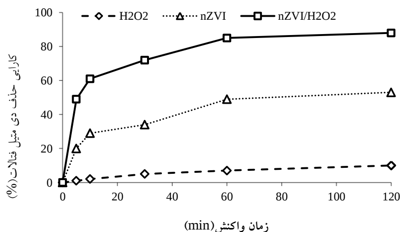
شکل ۵: تأثیر \text{nZVI.H}_2\text{O}_2 و \text{nZVI}/\text{H}_2\text{O}_2 در حذف دی‌متیل‌فتالات
