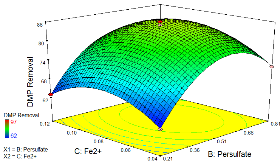
شکل ۳: تاثیر پرسولفات و تاثیر \text{Fe}^{2+} بر کارایی حذف DMP (غلظت ۵۰ mg/L)
