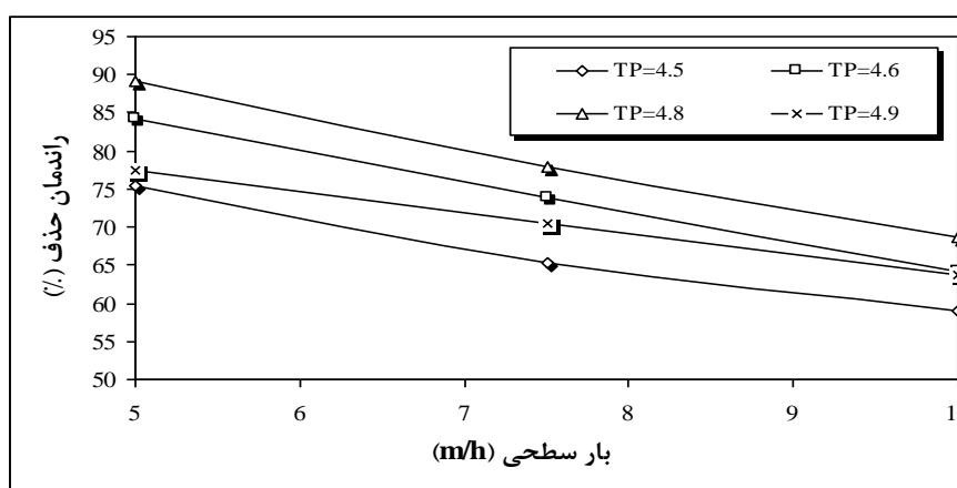
شکل ۶: میزان حذف فسفر کل در بارگذاری آلی و هیدرولیکی مختلف
