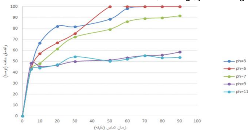
شکل ۲: راندمان حذف آلاینده ۲،۴ دی نیتروفلنل توسط نانو لوله کربن مغناطیسی شده از محلول آبی با تغییر pH
