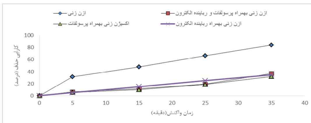
نمودار ۳: تعیین تأثیر پارامترهای مورد مطالعه بر کارایی حذف فورفورال از محیط
