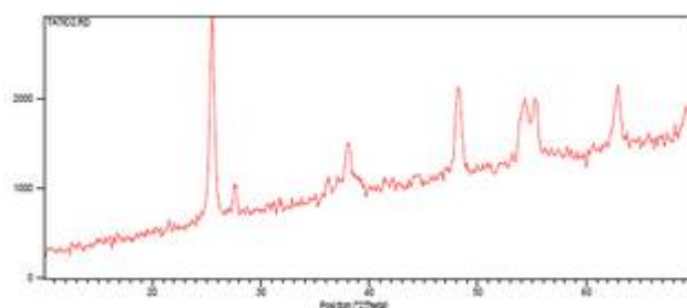
شکل ۱: طیف پراش اشعه ایکس (XRD) نانو کاتالیزور \text{TiO}_2
