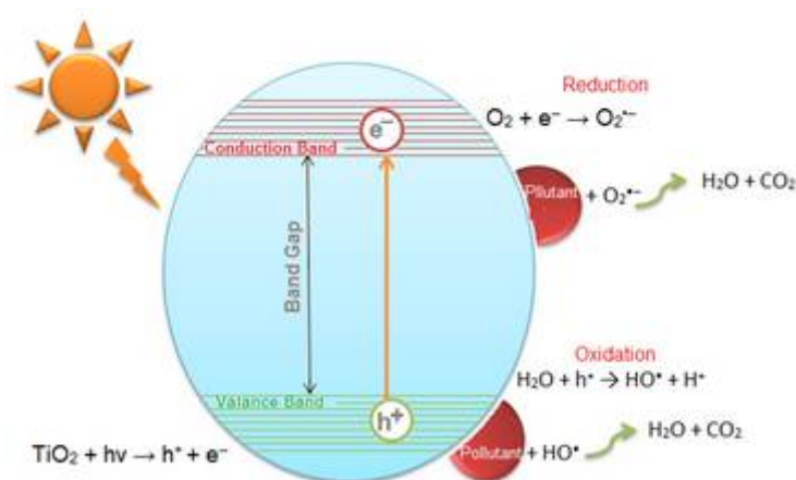
شکل ۱: مکانیسم تخریب فوتوکاتالیزوری به وسیله \text{TiO}_2 .
