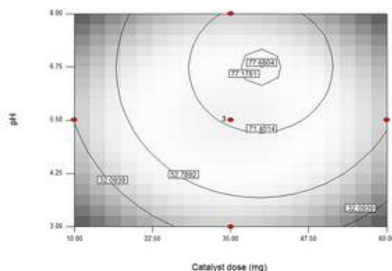
شکل ۷: تأثیر مقدار pH و مقدار کاتالیزگر بر کارایی حذف رنگ (در شرایط ثابت: غلظت محلول رنگی ۵۰ mg/L، دمای 25^\circ\text{C} ، مقدار کاتالیزگر ۲۷/۵۰ mg، pH=۳ و زمان ۲۰ دقیقه)
