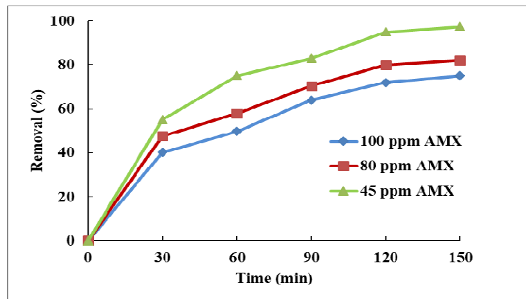
شکل ۵: تأثیر غلظت اولیه آنتی بیوتیک آموکسی سیلین بر کارایی سیستم (در شرایط nZVI = 0.2 g/L، H_2O_2 = 3\% ، pH = 3 و فرکانس ۱۳۰ کیلوهرتز)
