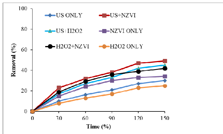
شکل ۶: تأثیر عوامل حذف در غیاب یک یا دو عامل (در شرایط AMX = 45 ppm، nZVI = 0.2 g/L، H_2O_2 = 3\% ، pH = 3 و فرکانس ۱۳۰ کیلوهرتز)
