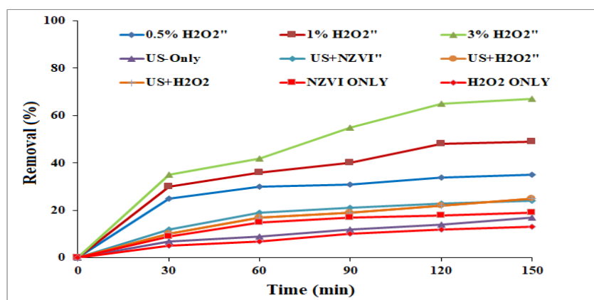
شکل ۷: کارایی سیستم در حذف COD (در شرایط AMX = 45 ppm، nZVI = 0.2 g/L، H_2O_2 = 3\% ، pH = 3 و فرکانس ۱۳۰ کیلوهرتز)
