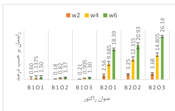
نمودار ۵: راندمان حذف کروم (VI) در هفته ۲، ۴ و ۶ در غلظت ۳۵۰ mg/kg
