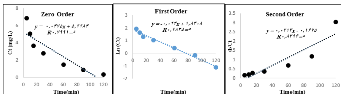
شکل ۹: بررسی مدل سینتیکی درجه صفر، درجه اول و درجه دوم در فرایند (غلظت سفتریآکسون ۱۰ mg/L، pH=۳، اولیه، دوز کاتالیست ۲ g/L، زمان ۵-۱۲۰ دقیقه)
