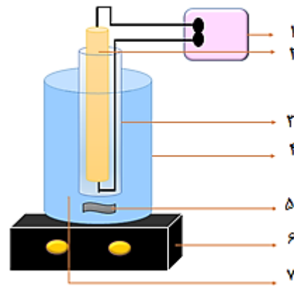
شکل ۱: شماتیکی از راکتور مورد استفاده در این مطالعه (۱: منبع انرژی، ۲: لامپ UV، ۳: پوشش کوارتزی، ۴: ظرف شیشه ای، ۵: مگنت، ۶: میکسر، ۷: محلول آنتی بیوتیک)
