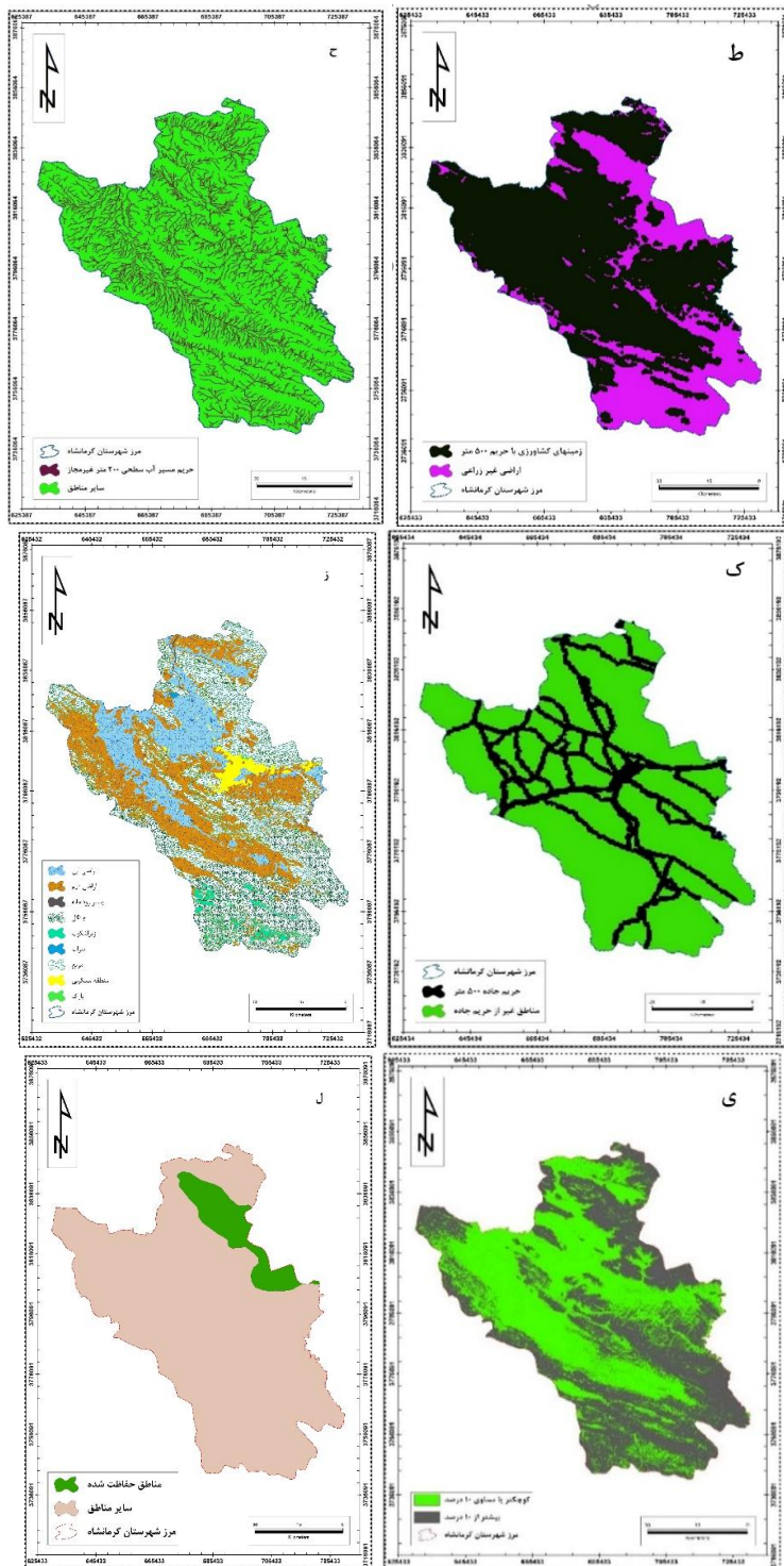
شکل ۲: لایه‌های اطلاعاتی مورد استفاده در انتخاب محل مناسب دفن پسماندهای جامد شهری کرمانشاه؛ الف) فاصله از گسل، ب) فاصله از فرودگاه، ج) نفوذپذیری خاک، د) عمق آب زیرزمینی، ه) فاصله از زمین های کشاورزی، و) خطوط نیرو، ز) کاربری اراضی، ح) آب های سطحی، ط) پوشش گیاهی و باغی، ی) شیب، ک) فاصله از جاده؛ ل) فاصله از مناطق حفاظت شده
